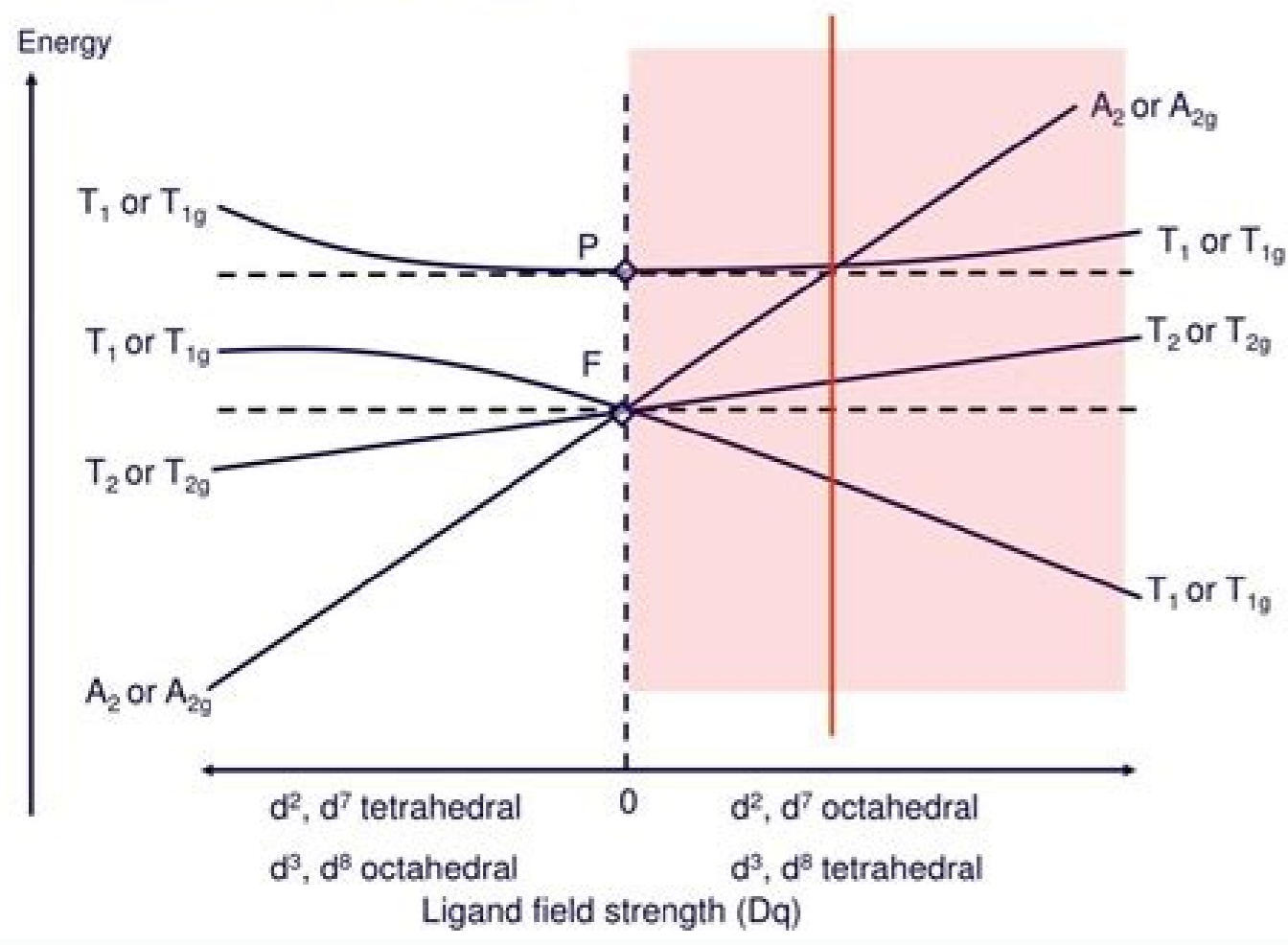
Orgel diagram for d^2 , d^3 , d^7 , d^8 ions
